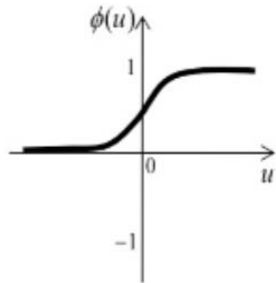
sigmoid function
